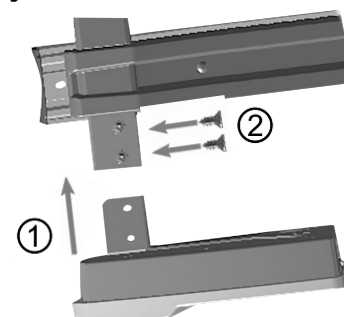
Bild 2: Montage Rückleuchten
