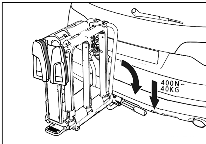
Bild 10: Schließen des Schnellverschlusses
