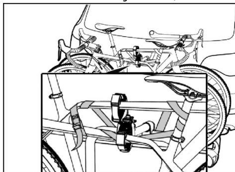
Bild 18: Sicherheitsgurt anlegen
