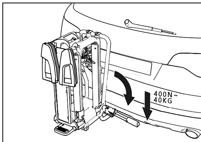
Figura 10: Chiusura della chiusura rapida
