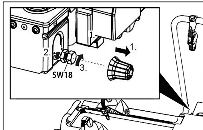
Figure 13: Réglage de la fermeture rapide
