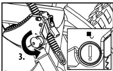
Figure 17 : Fixer le support de cadre
