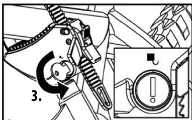
Bild 17: Rahmenhalter befestigen
