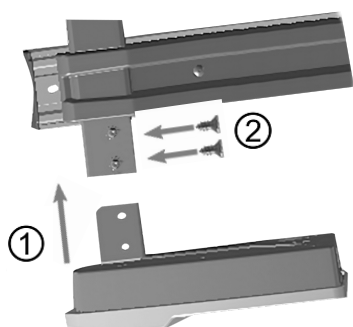
Figura 2: Montaggio delle luci posteriori
