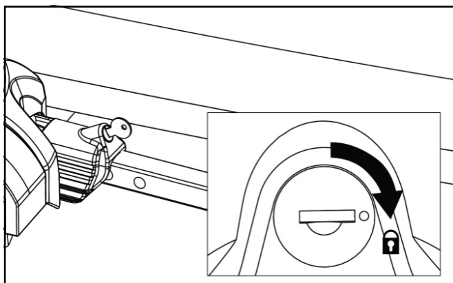
Bild 12: Abschließen des Schnellverschlusses
