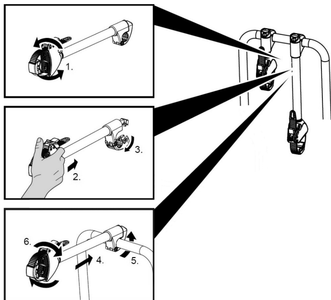
Figura 7: Montaggio del supporto del telaio
