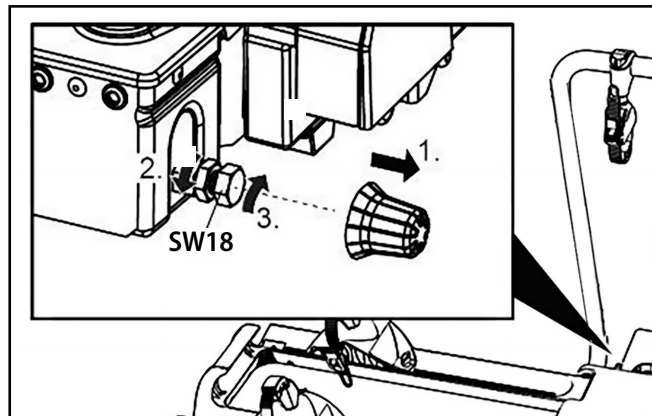
Bild 13: Einstellen des Schnellverschlusses
