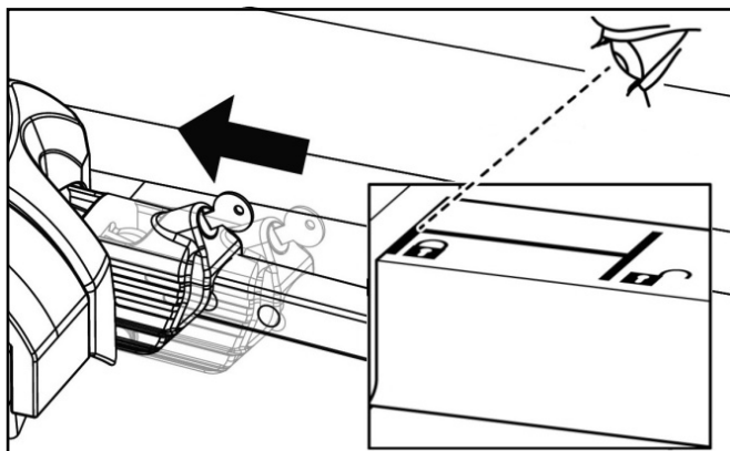
Bild 11: Verriegeln des Schnellverschlusses
