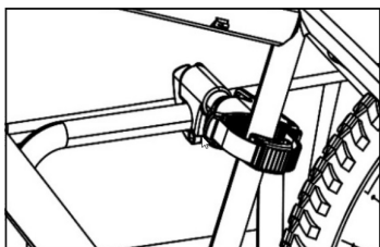
Bild 16: Rahmenhalter einstellen
