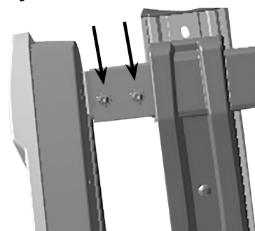
Bild 3: Montage Rückleuchten
