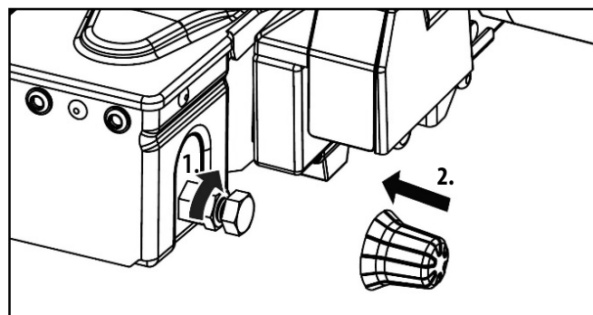
Figure 14: Réglage de la fermeture rapide
