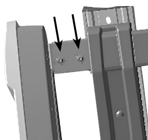
Figure 3 : Montage des feux arrière
