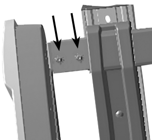
Figura 3: Montaggio delle luci posteriori
