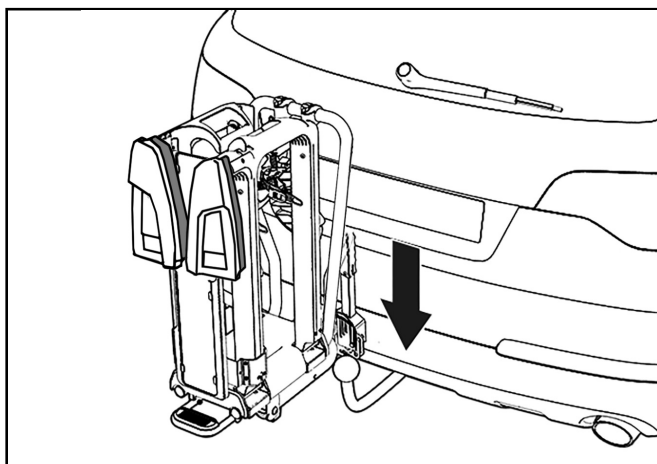
Figure 9: Mise en place du support sur l'attelage de remorque
