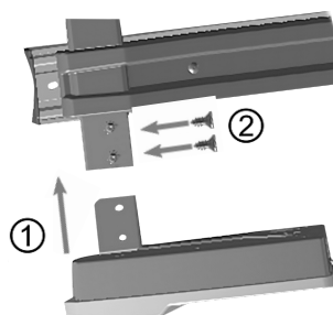
Figure 2 : Montage des feux arrière
