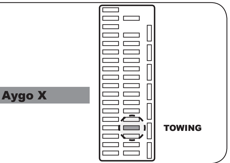
Sicherungskasten fusebox
