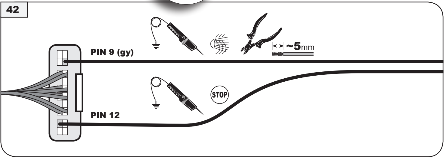
Fahrzeuge Stecker 18 pin bu car socket 18 pin bu
