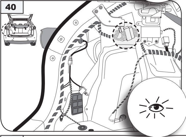
Fahrzeuge Stecker 18 pin bu car socket 18 pin bu
