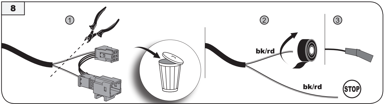
E-Satz Stecker e-kit socket
