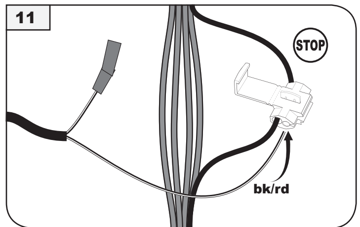
E-Satz bk/rd → kabel Fahrzeug (STOP) e-kit bk/rd → cabel car
