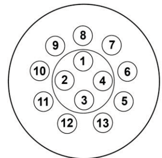
Collegamento dei cavi alla presa a 13 poli
