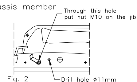
Fig. 2 Drill hole \phi 11\text{mm}
